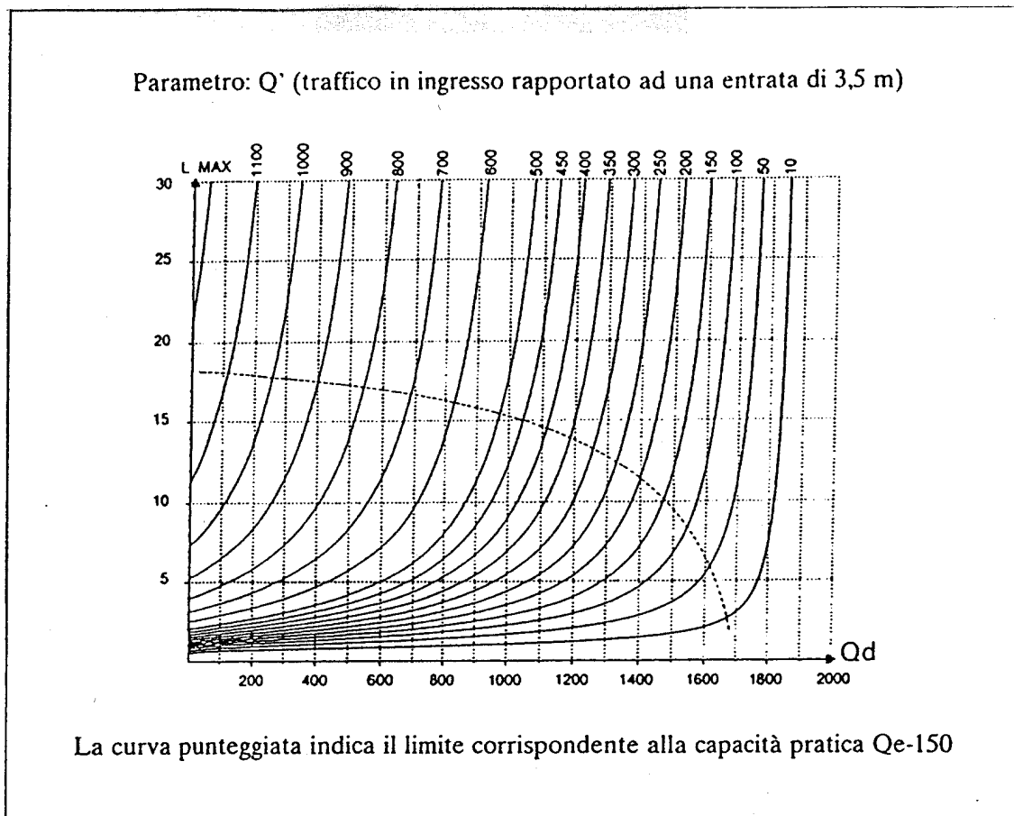
Fig. 3 – 99° percentile del numero di veicoli in attesa su un braccio di rotatoria
