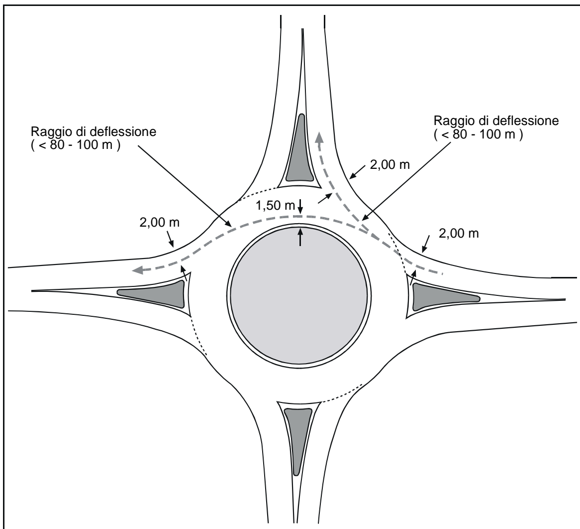
Fig. 13 – Deflessione della rotatoria
