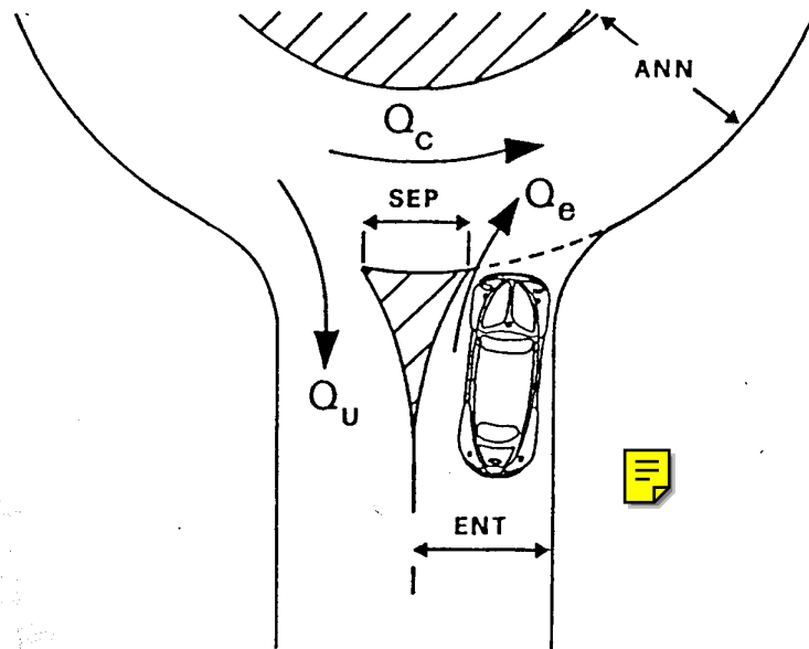
Fig. 1 – Caratteristiche geometriche e di traffico di una rotatoria
