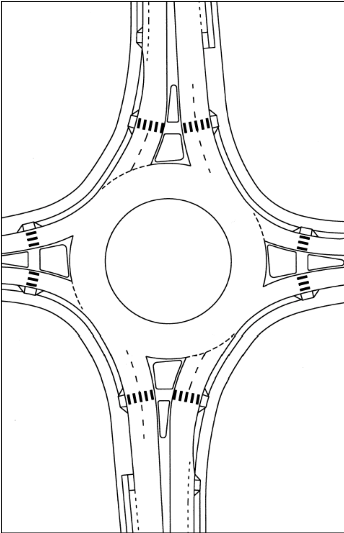
Figura 9: Esempio di rotonda con ingressi allargati (“scampanati”).
