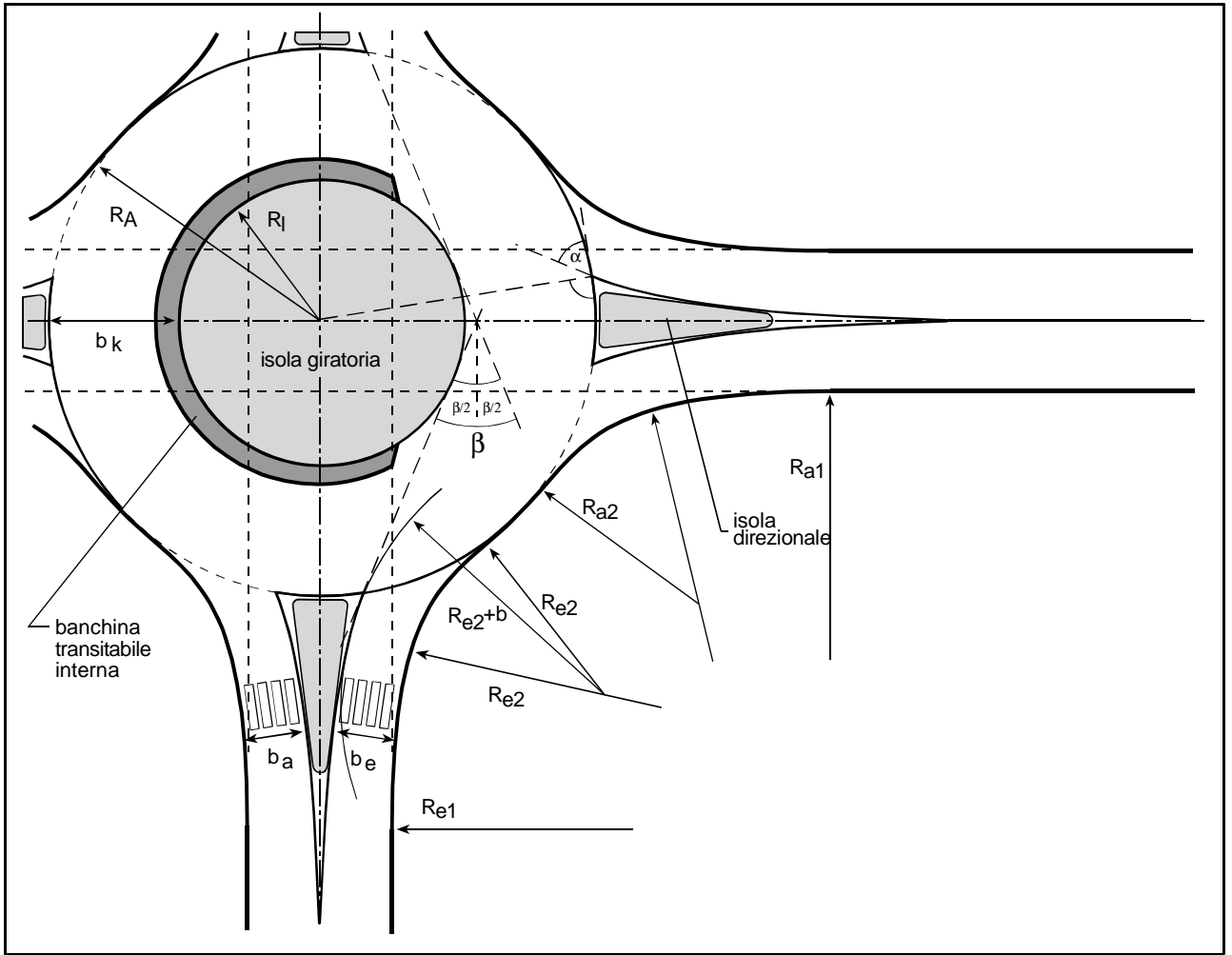
Fig. 14 – Elementi di progetto e tipizzazione delle rotatorie
