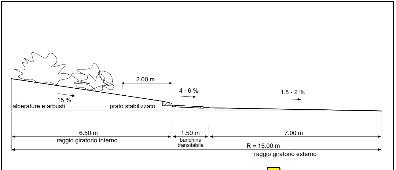
Fig. 11 – Isola centrale di rotondina compatta
