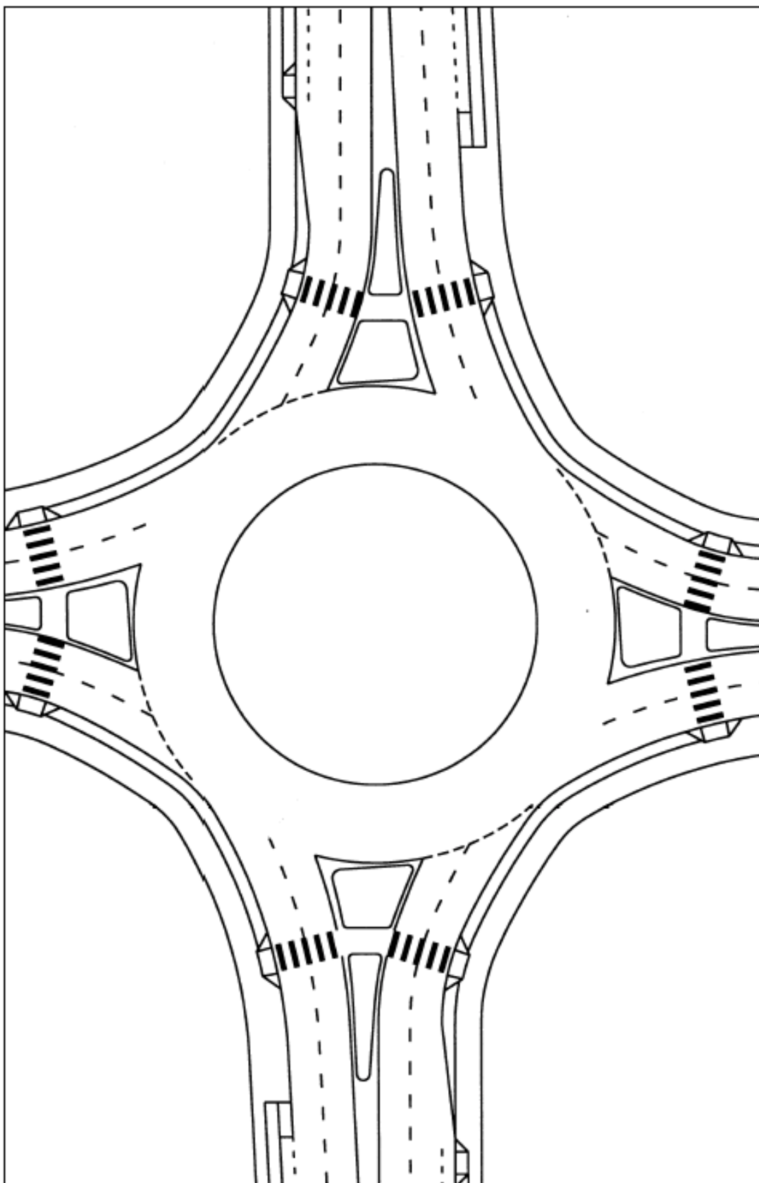
Figura 8: Esempio di rotonda urbana a doppia corsia
