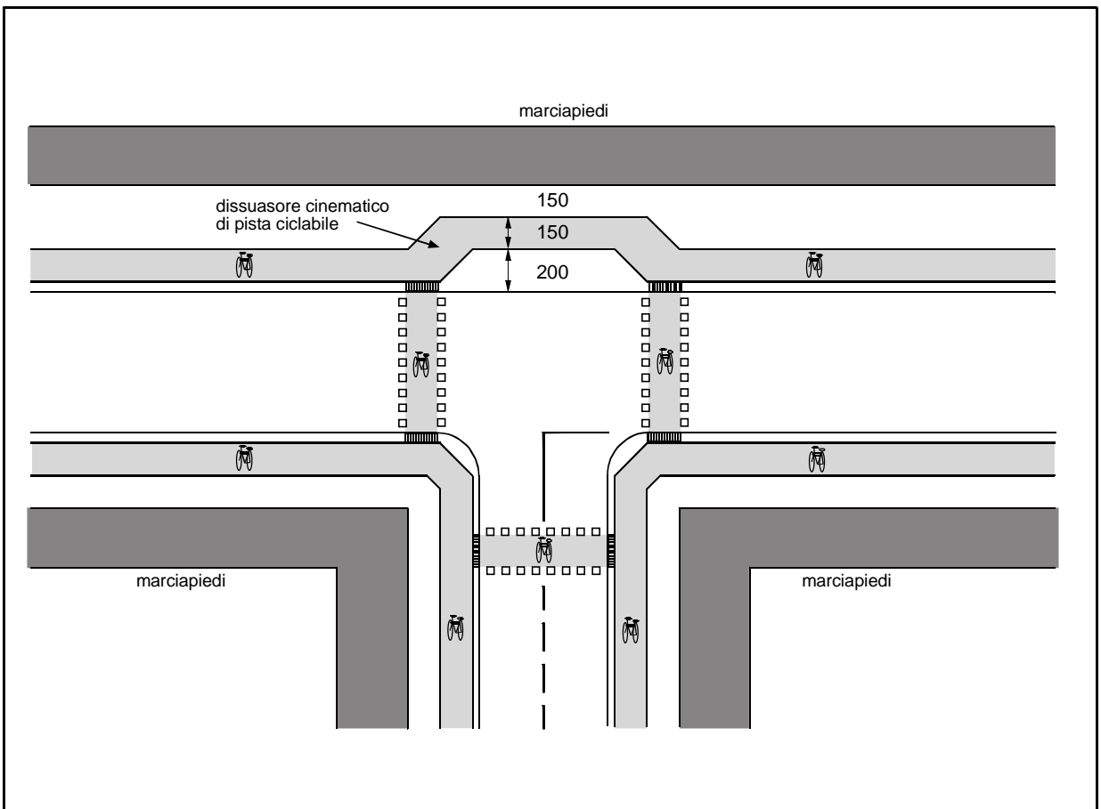
Fig. 19 – Attraversamento promiscuo pedonale e ciclabile
