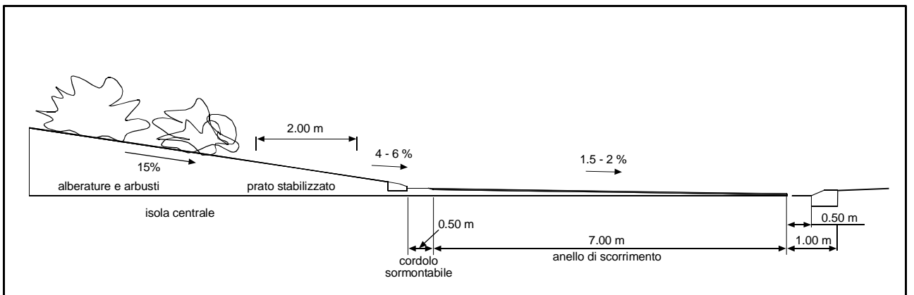
Fig. 12 – Isola centrale per minirotatoria
