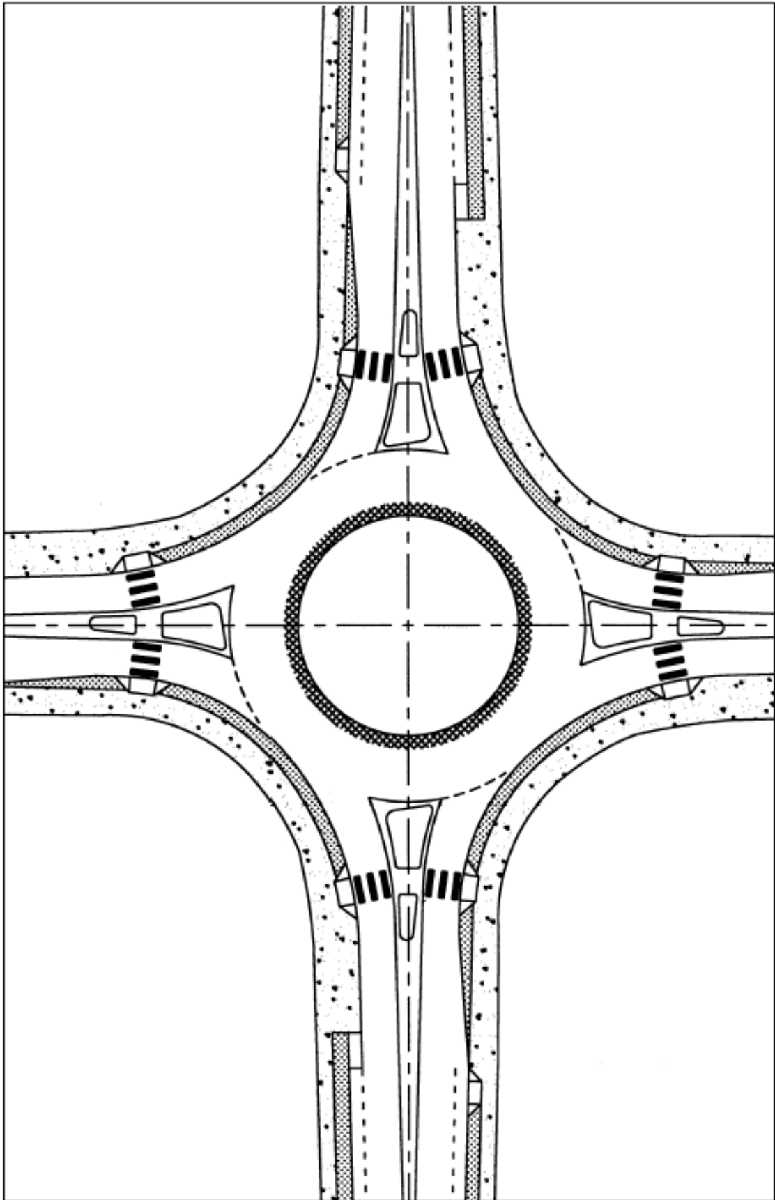
Figura 7: Esempio di rotatoria urbana a singola corsia.
