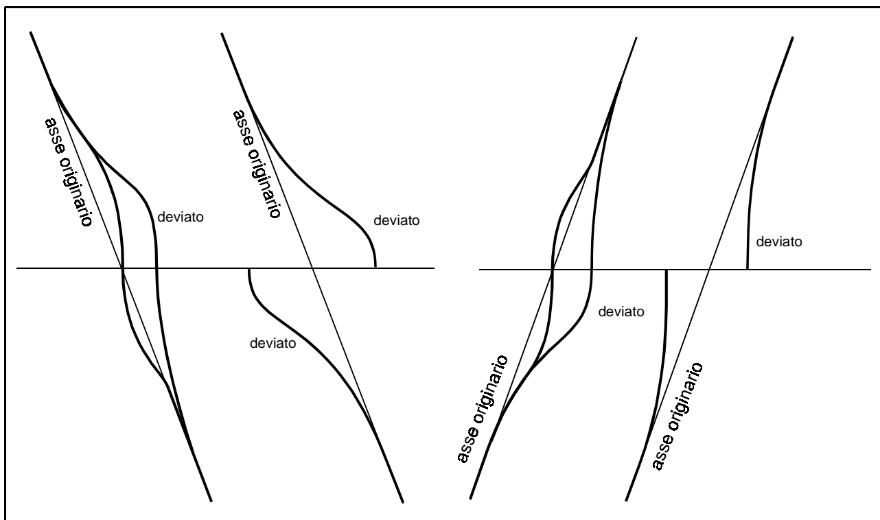
Fig. 7 – Rettifica d'asse della secondaria
