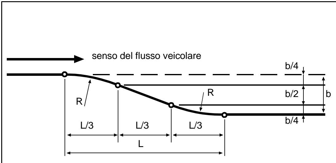
Fig. 16 – Elementi della linea di ciglio
