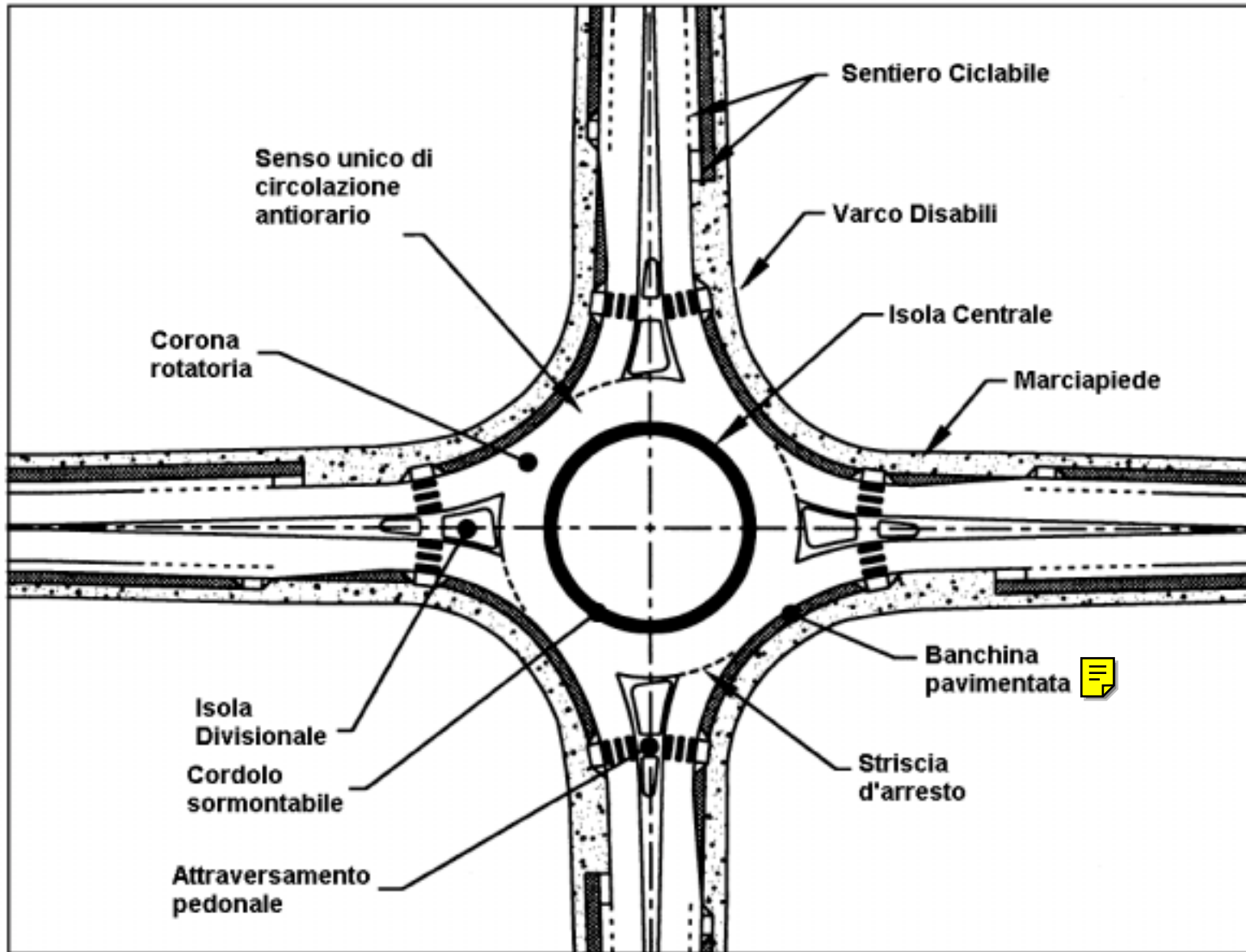
Figura 5: elementi caratteristici delle rotatorie di piccolo diametro.
