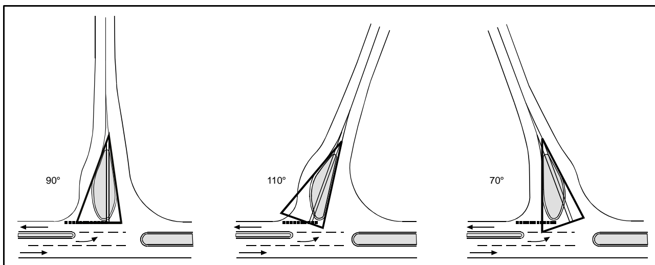
Fig. 8 – Angolazioni del triangolo di costruzione
