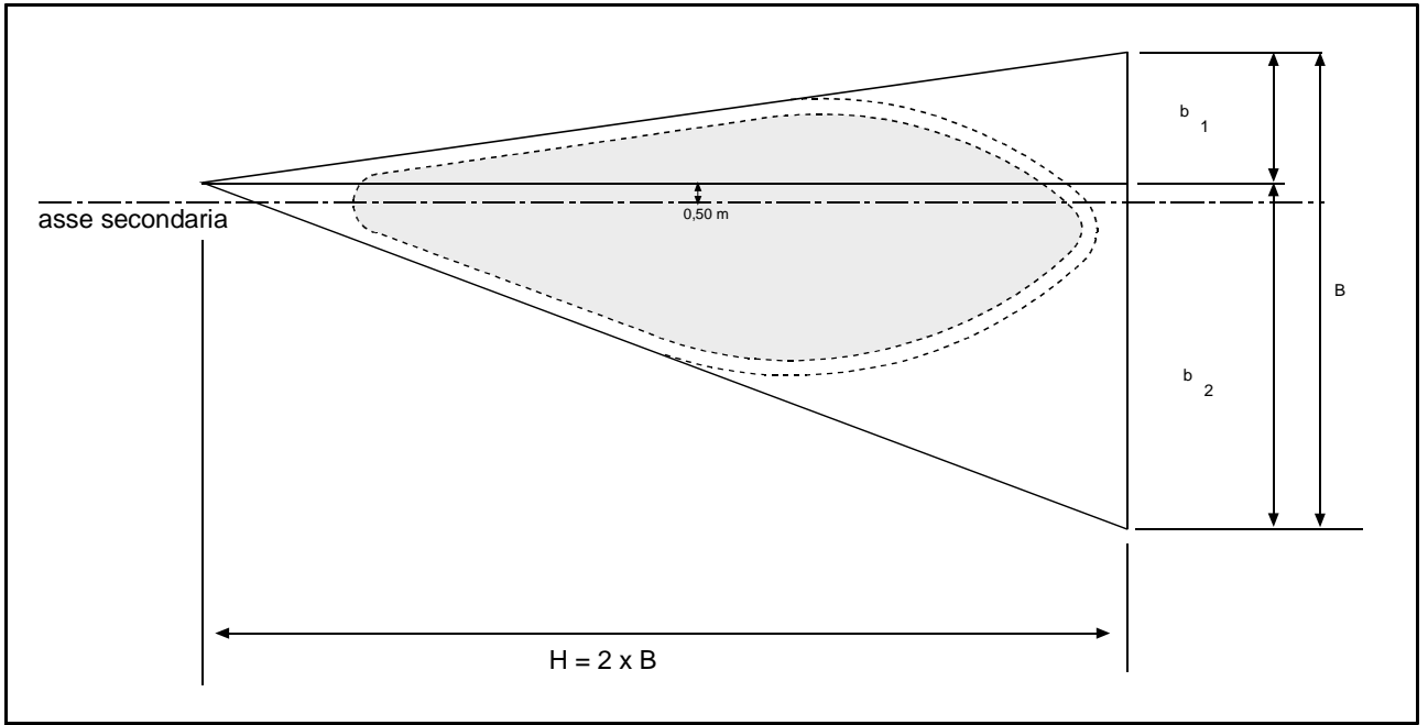
Fig. 9 – Triangolo di costruzione
