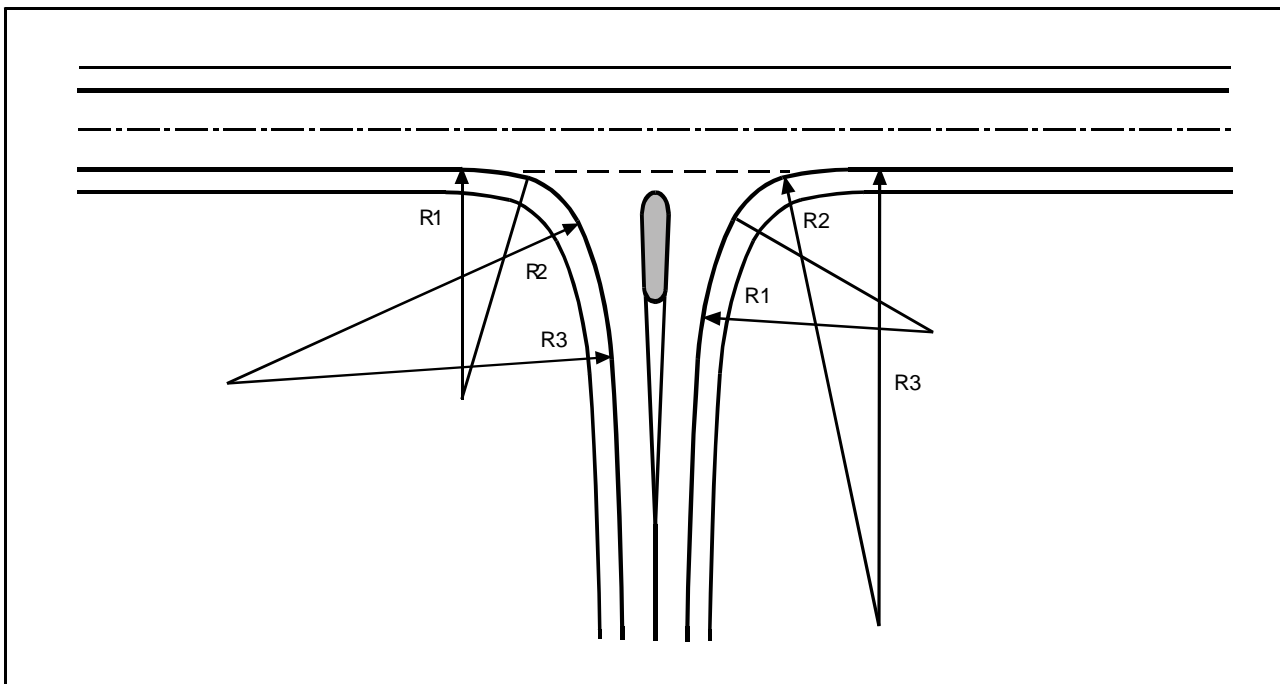
Fig. 17 – Tricentrica di ciglio
