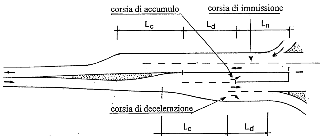
Fig. 1- Elementi delle corsie di decelerazione e di accumulo
