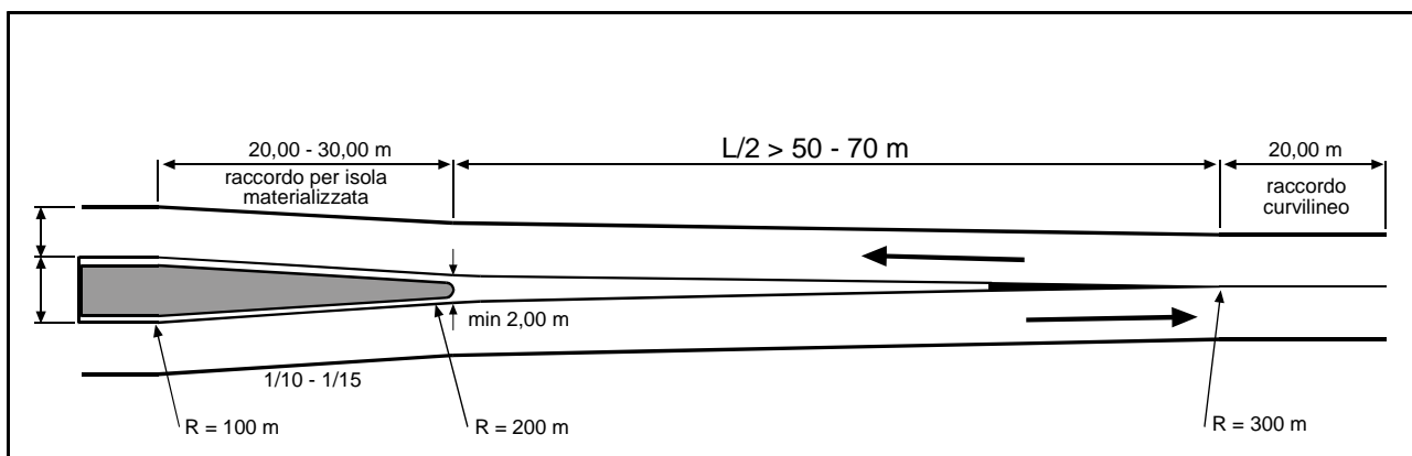
Fig. 5 – Tratto iniziale di isola di mezzeria
