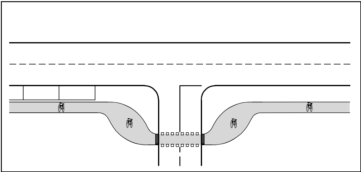
Fig. 18 – Arretramento protetto di pista ciclabile
