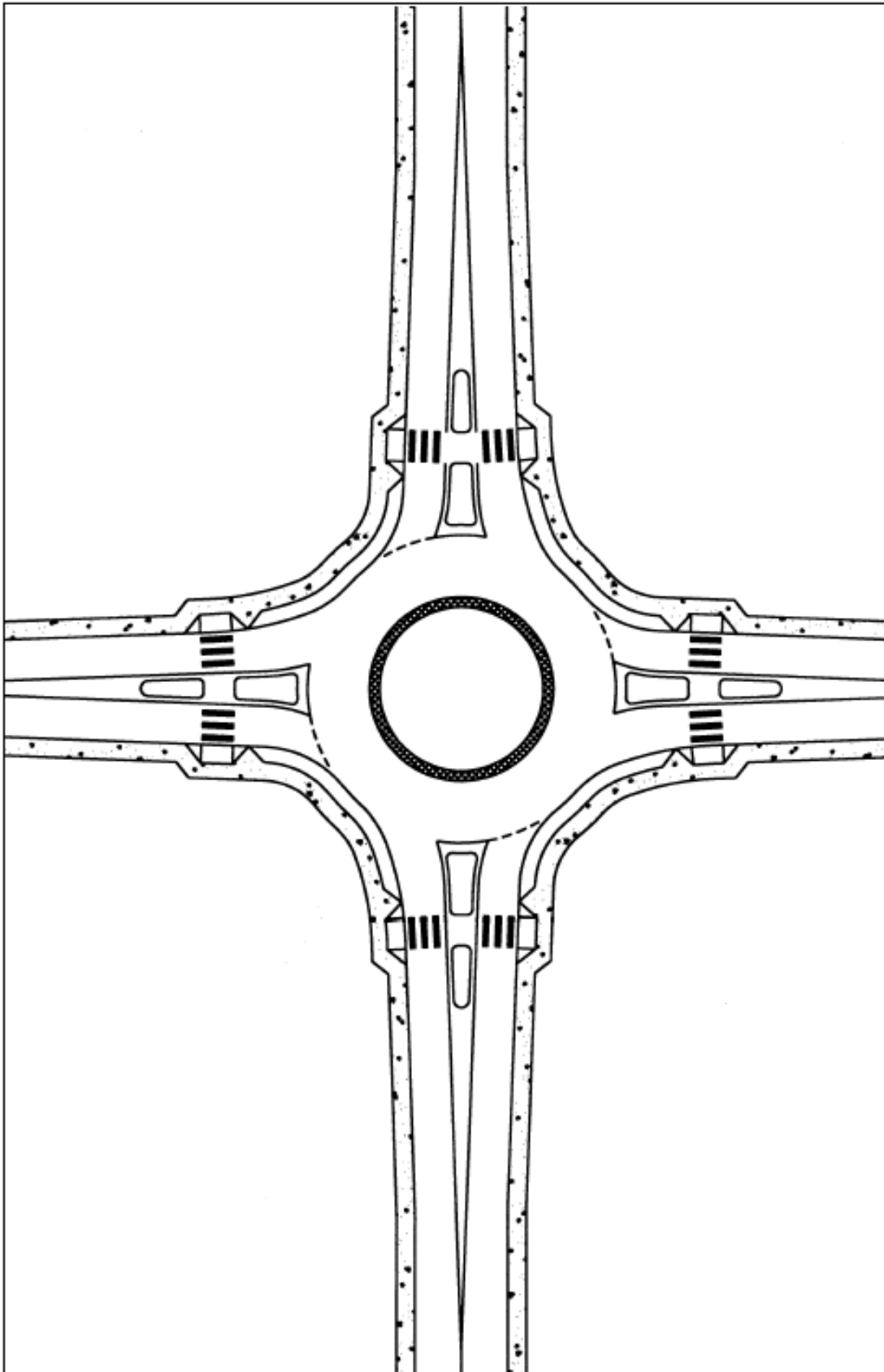
Figura 6: Esempio di rotonda urbana compatta.
