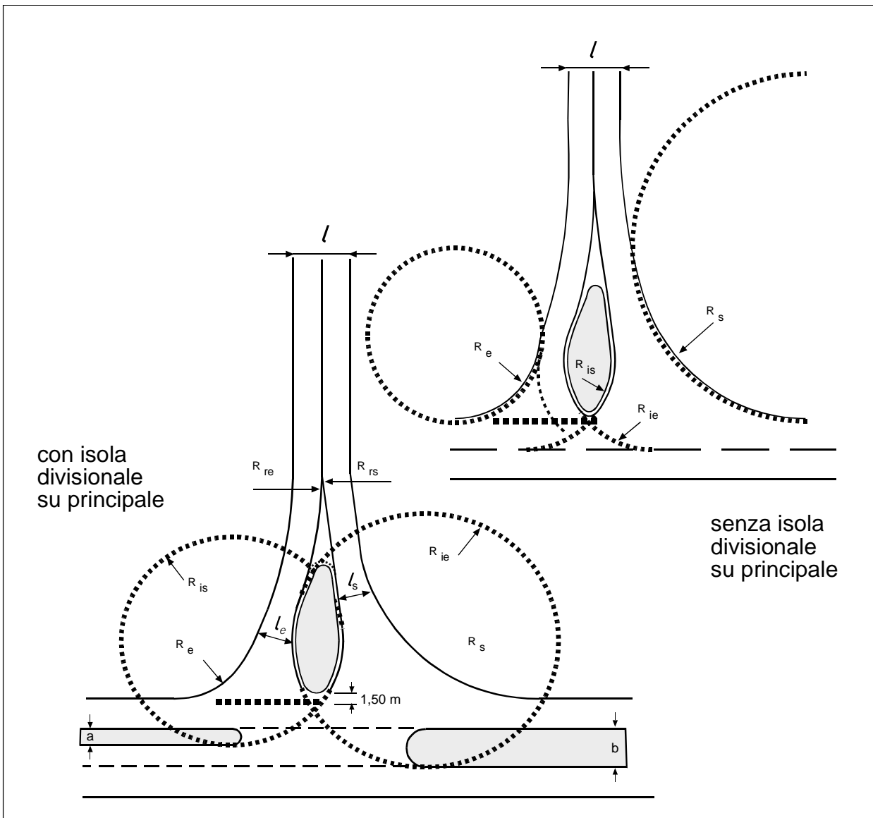
Fig. 10 – Tracciamento isola a goccia
