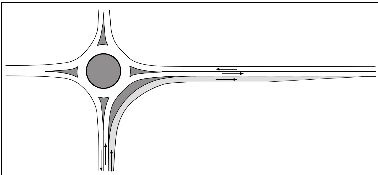
Fig. 15 – Rotatoria potenziata con svolta diretta
