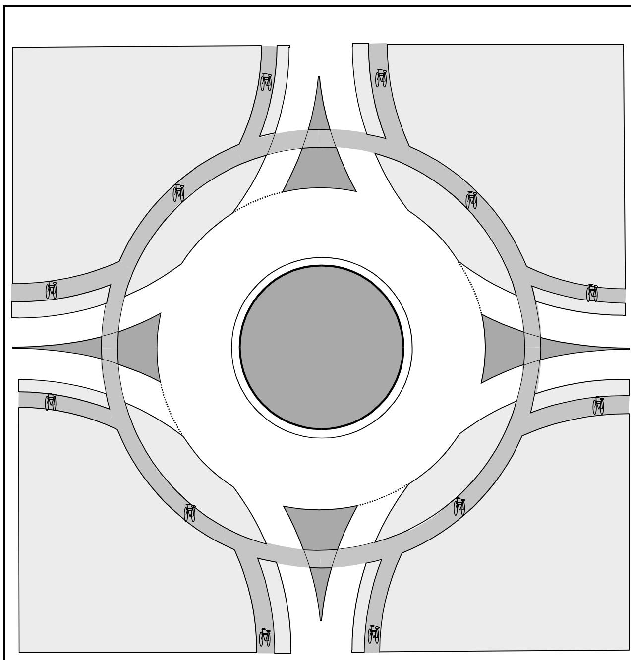
Fig. 21 – Rotatoria ciclabile esterna
