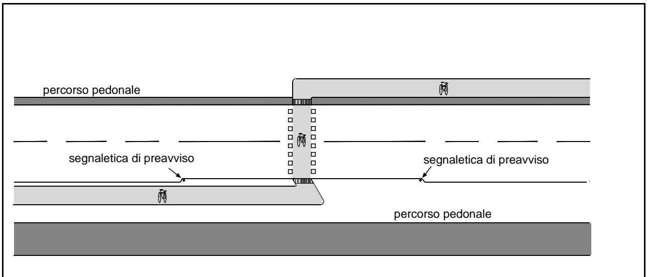
Fig. 20 – Attraversamento specializzato per pista ciclabile in arretramento da incrocio
