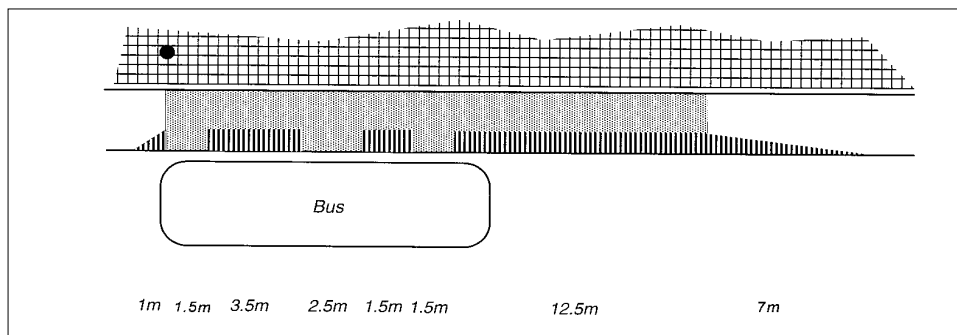
Fig. A1.3.5 - Esempio di sistemazione all'intersezione tra pista ciclabile e area di fermata dei mezzi pubblici Vejdirektoratet, 1993.
